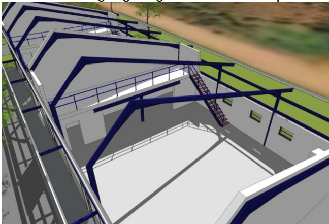
Vorher - Bauplan
